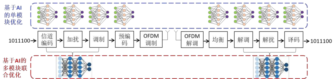
图 12： 物理层信号处理中基于 AI 的单模块优化和基于 AI 的多模块联合优化示例
