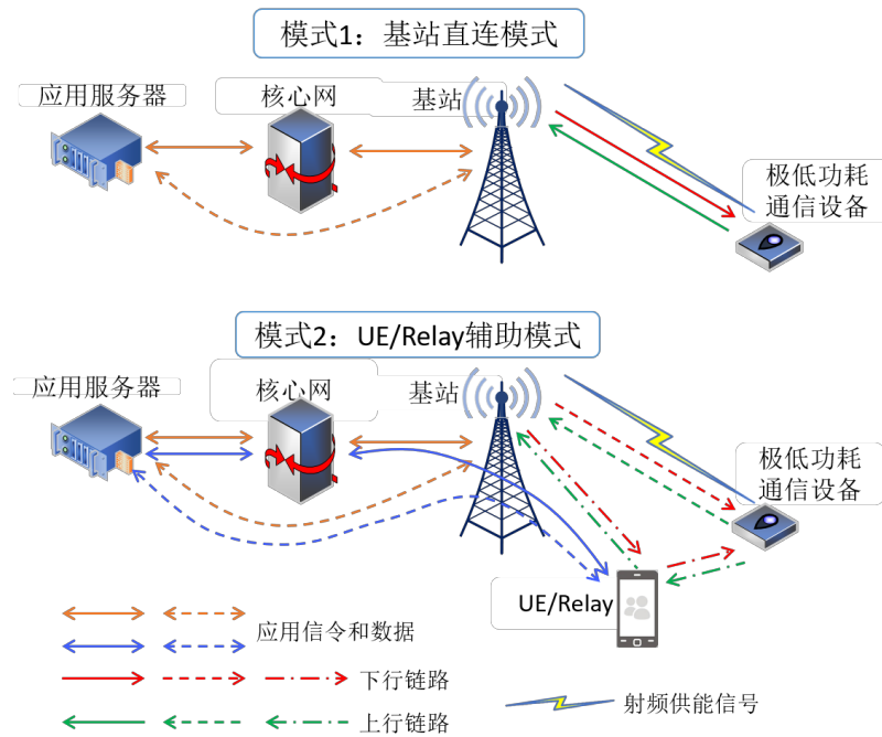
图 19：极低功耗通信与蜂窝通信融合的网络架构
