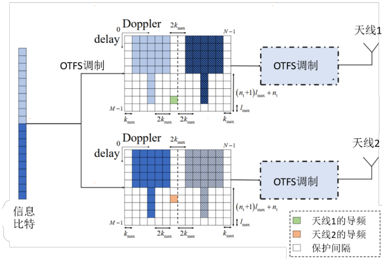
图 28：OTFS-MIMO 开环预编码
